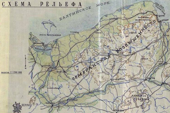
Схема рельефа Померанской возвышенности.
